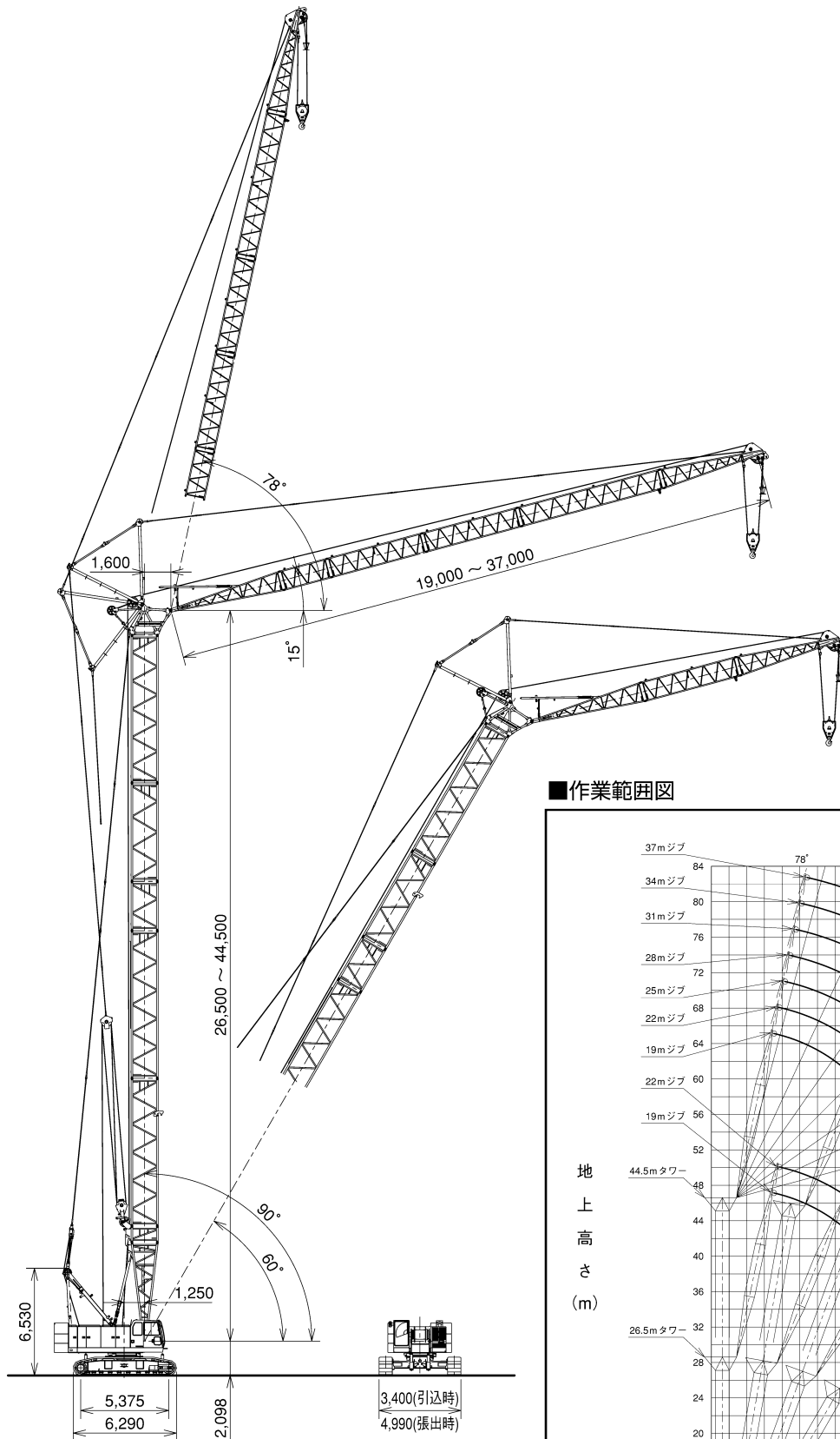
■全体図 (単位 mm) ( \frac{1}{400} )
